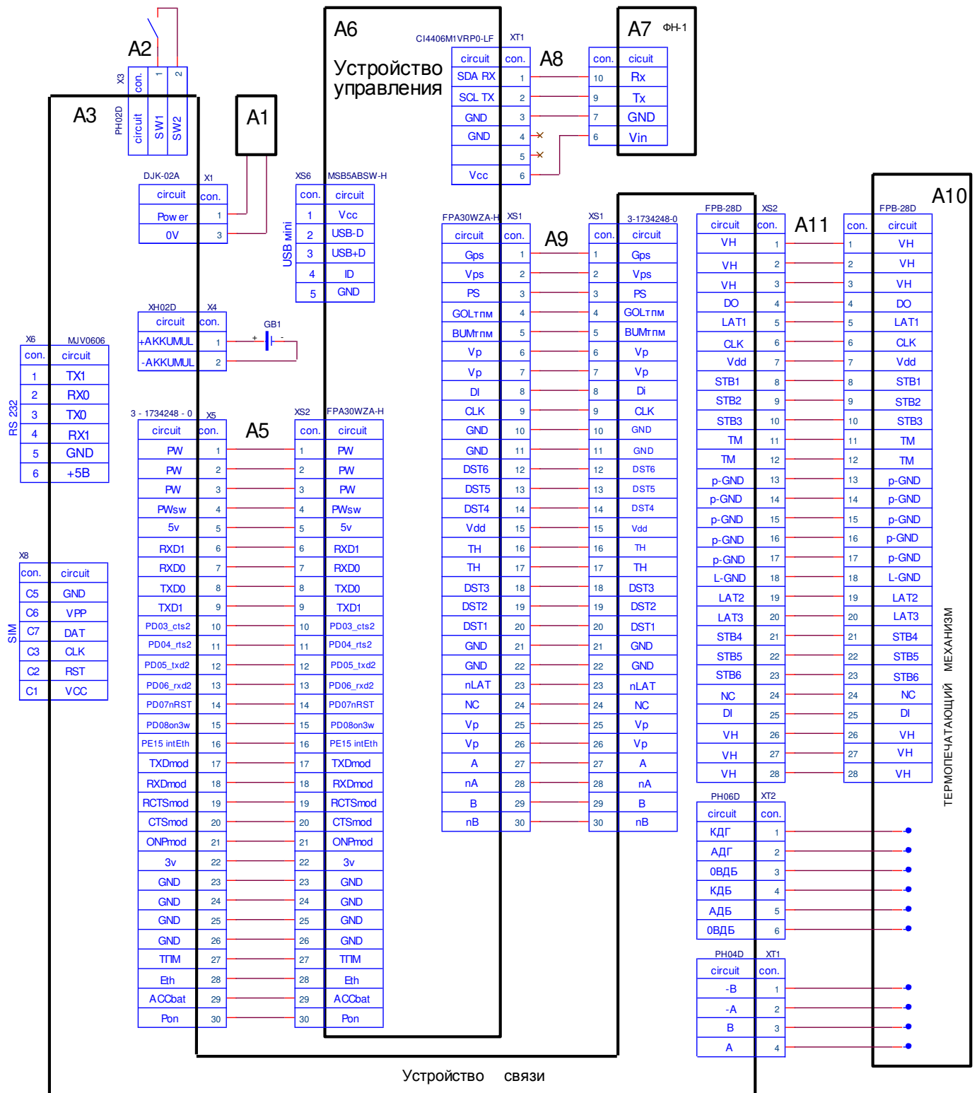
Схема соединений
