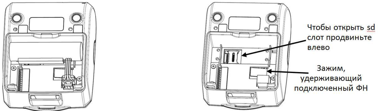
Рис.1 Внутренний отсек ККТ
