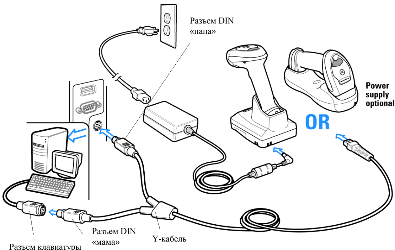
Рисунок 6-1 Подключение Keyboard Wedge с Y-образным кабелем
